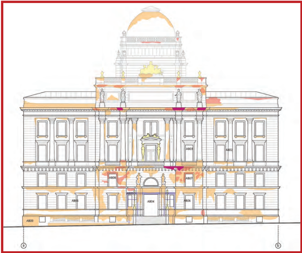
Fotografija 43. Oštećenja na frontalnoj fasadi (&+A) – Ammar Akšamija, Dženis Avdić i / “Arhiv Akšamija” Sarajevo. 2021)
