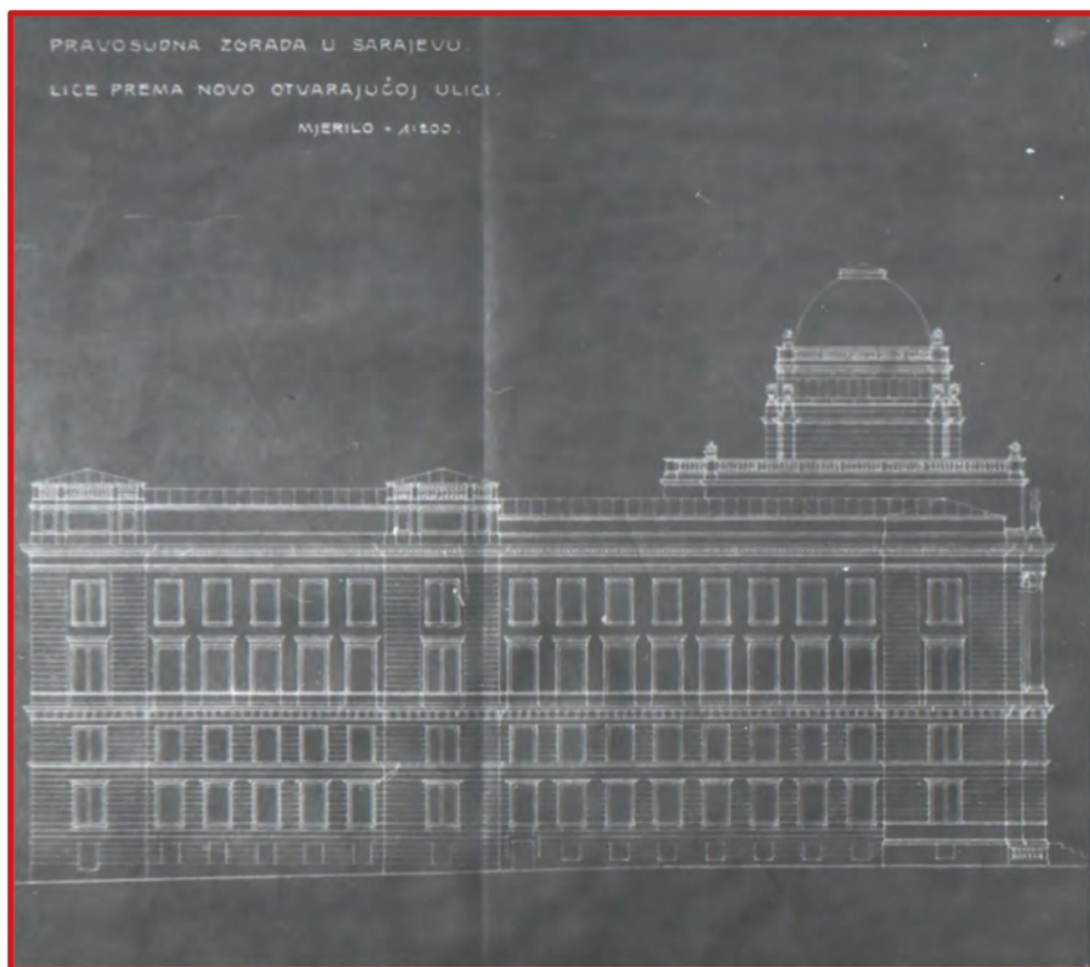
Fotografija 23. Plan Pravosudne palate – Lice prema Jadranskoj ulici (&+A) – Ammar Akšamija, Dženis Avdić i / “Arhiv Akšamija” Sarajevo, 2021)
