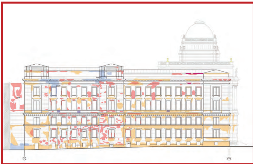
Fotografija 44. Oštećenja na podužnim fasadama i dvorištu (&+A) - Ammar Akšamija, Dženis Avdić i / “Arhiv Akšamija” Sarajevo, 2021)
